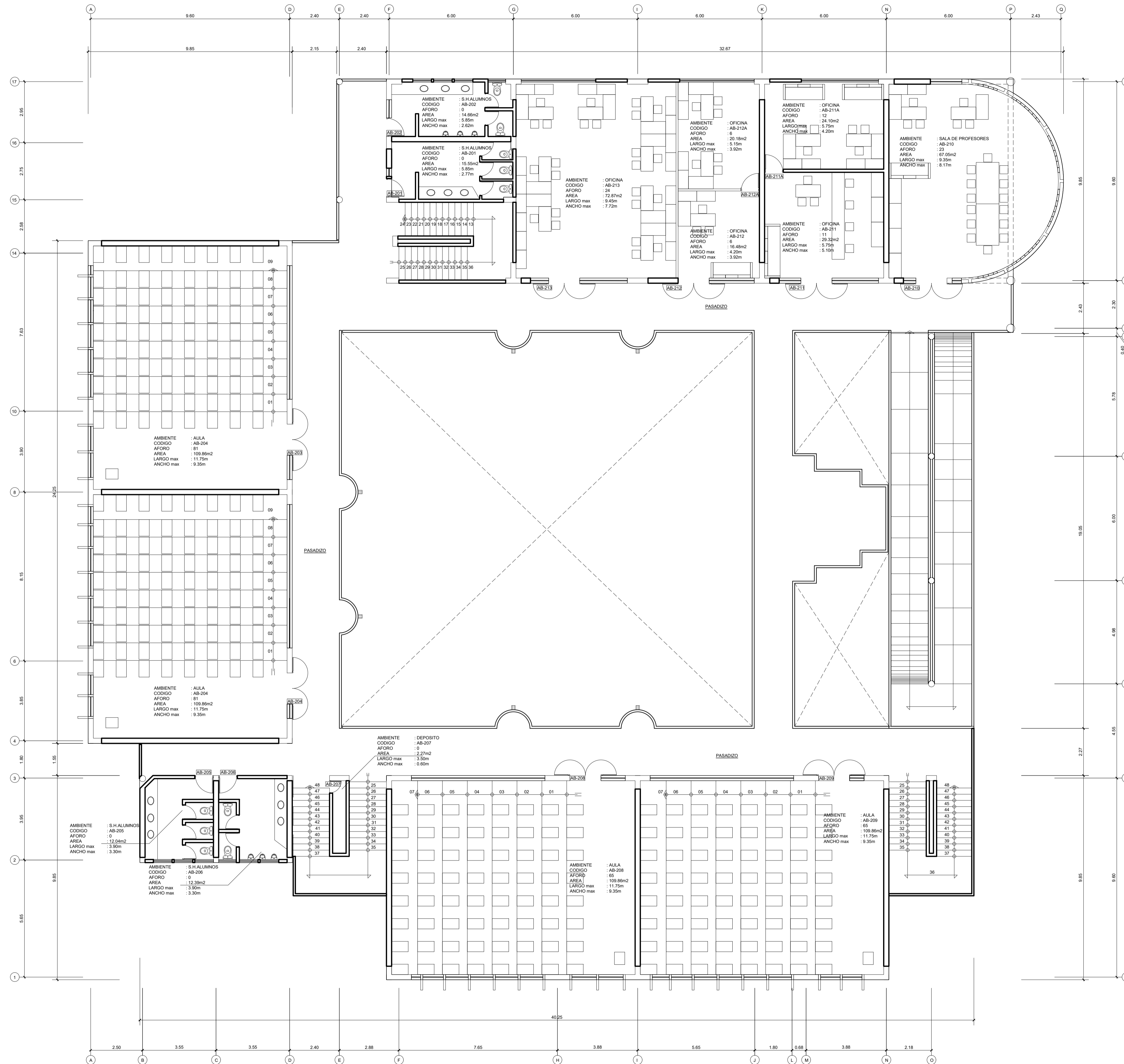
SEGUNDA PLANTA AREA TECHADA = 1123.21m 2 AFORO = 374 ESCALA 1:100
